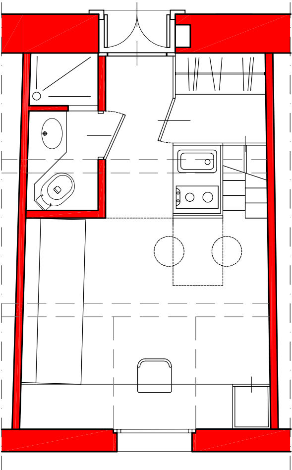
PIANTA SOPPALCO
